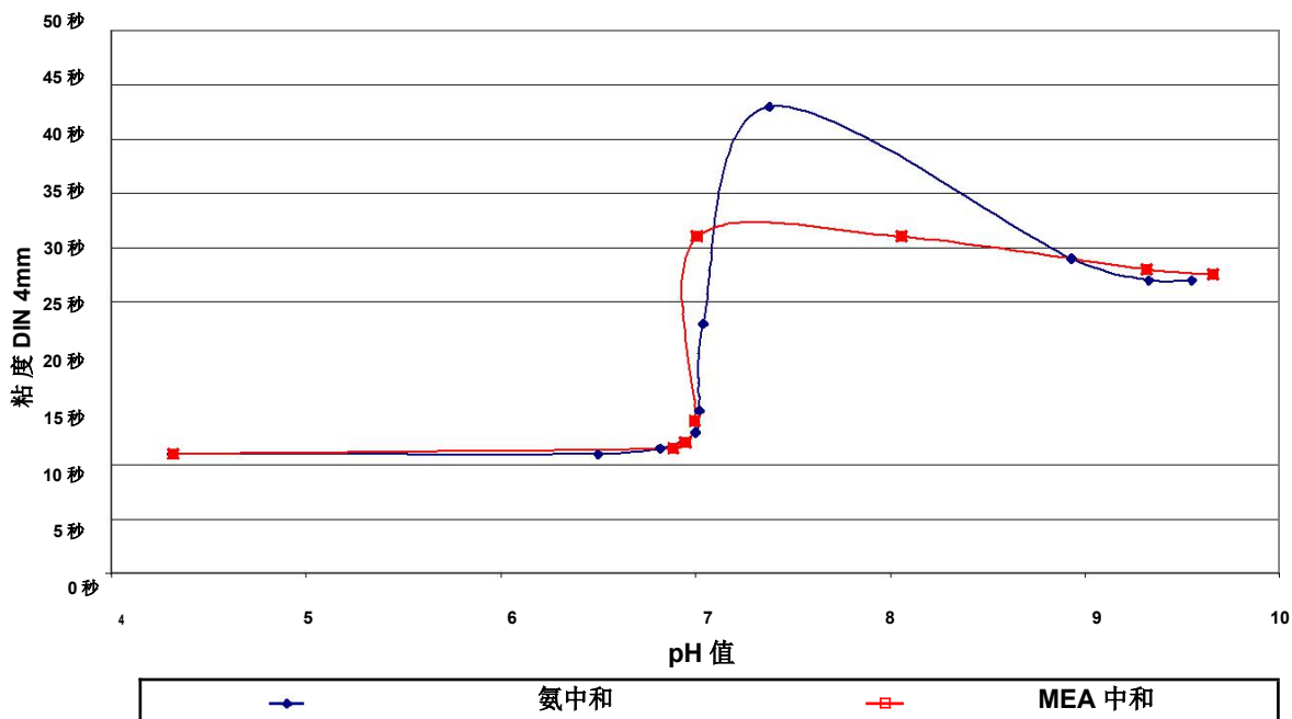
PAC 281中和后溶液的粘度 (保持固体含量10.5%)
